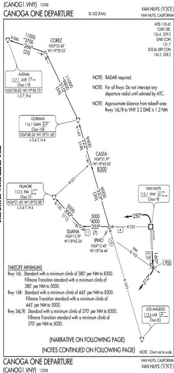
(CANOG1.VNY) 12208 CANOGA ONE DEPARTURE SL-552 (FAA) VAN NUYS (VNY) VAN NUYS, CALIFORNIA
